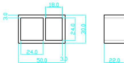
CORTE A-A'
