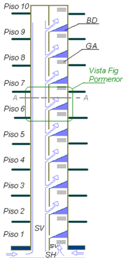
Esquema de elevação
